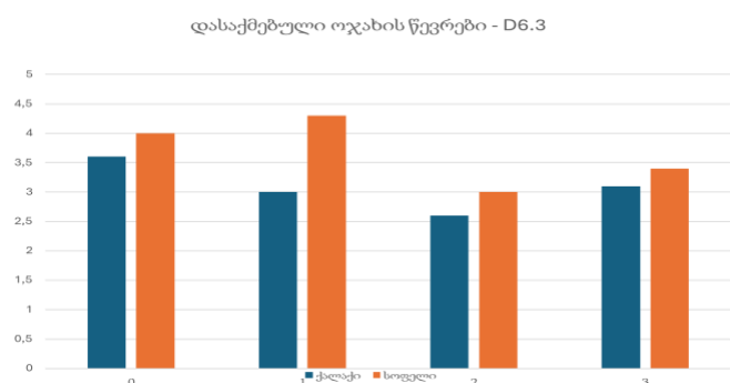
ჰისტოგრამა D6.3
