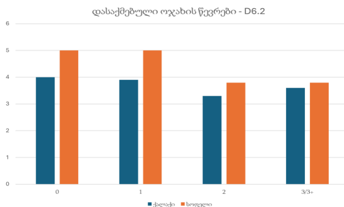
ჰისტოგრამა D6.2
